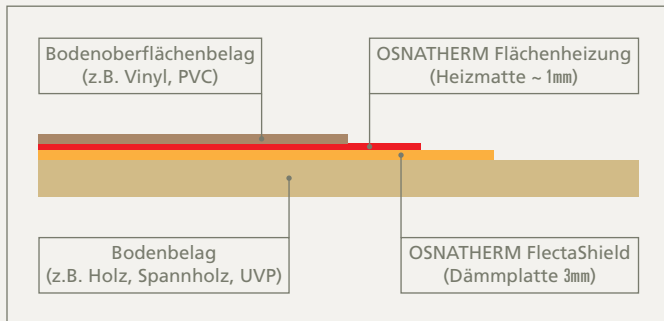
Schichtenansicht der Flächenheizung
